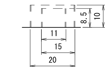
側面ノックアウト 詳細 (1/1)
